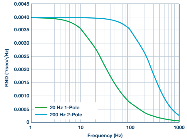
图4. 使用滤波器时的ADXRS290噪声密度
