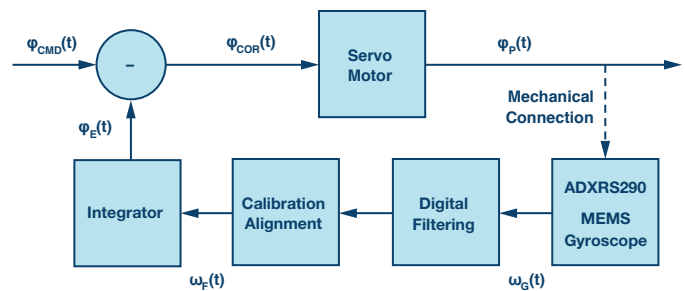
图1. 运动控制系统架构示例
